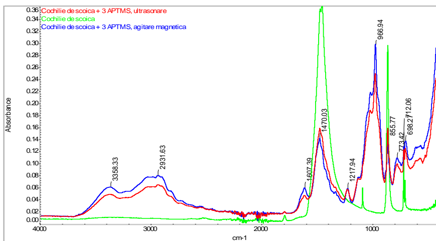
Fig.8. Spectrele FT-IR ale cochiliei de scoici nefuncționalizată și funcționalizată cu 3-APTMS prin cele două metode.
