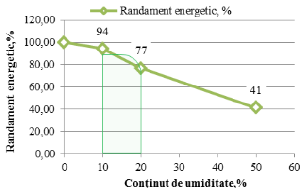
Fig. 3. Variația randamentului energetic în cazul biomasei lemnoase de frasin.
