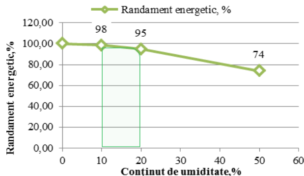
Fig.4. Variația randamentului energetic în cazul biomasei lemnoase de paltin de munte.
